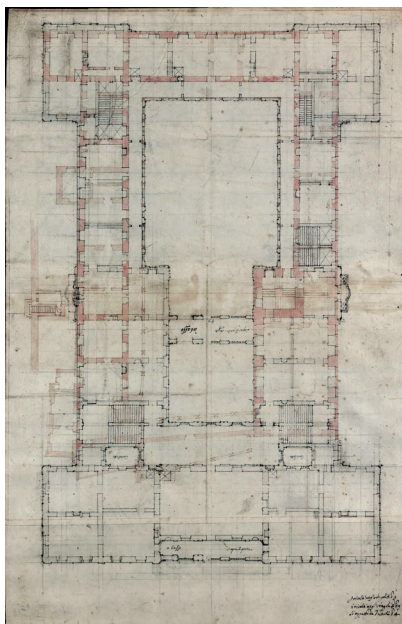
Martinelliho návrh přízemí a prvního patra zámku ve Slavkově. Mezi lety 1694–1696. (převzato z: A. Scotti Torsini, Domenico Martinelli – architetto ad Austerlitz. I disegni per la residenza di Dominik Andreas Kaunitz (1691–1705), 2006.)
