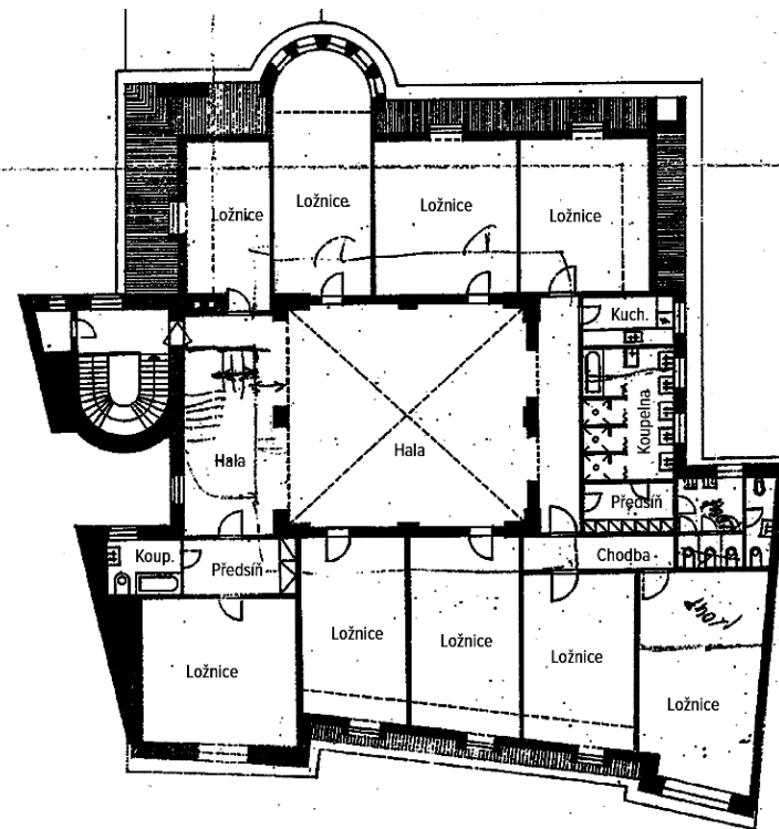
Návrh nového podkroví, plán přestavby z roku 1968. (převzato z J. Eliáš, Stavebně historický průzkum vily Löw-Beer , 2011)
