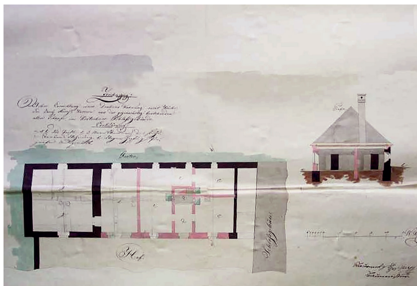
Návrh přestavby hospodářského traktu zámku, vypracovaný v roce 1828 stavitelem Neuwerthem. (MZA v Brně) Zeleně vyznačená část okolo půdorysu objektu představuje zámeckou zahradu, šedá vpravo pak budovu zámku.
