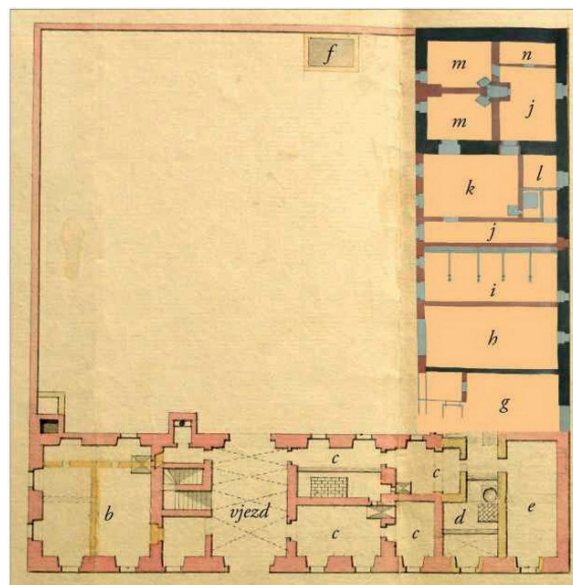
Plán zámku upravený autorem pro potřeby tohoto textu. (MZA v Brně, archiv autora) V dolní části je výkres mistra Zeyssla, vypracovaný pro stavbu realizovanou v letech 1792–1795. Vpravo nahoře je stavební dispozice přestavby hospodářského traktu na byt drába a vězení, kterou kapitule v roce 1828 představil stavitel Neuwerth. Plán 1792–1799: b) kancelář, c) byt důchodního, d) prádelna, e) mandlovna, f) hnojník. Plán 1828: g) skladiště purkrabího, h) kůlna pro vozy, i) stáj pro pět koní, j) chodba, k) pokoj drába, l) kuchyně, m) vězení, n) kancelář drába.
